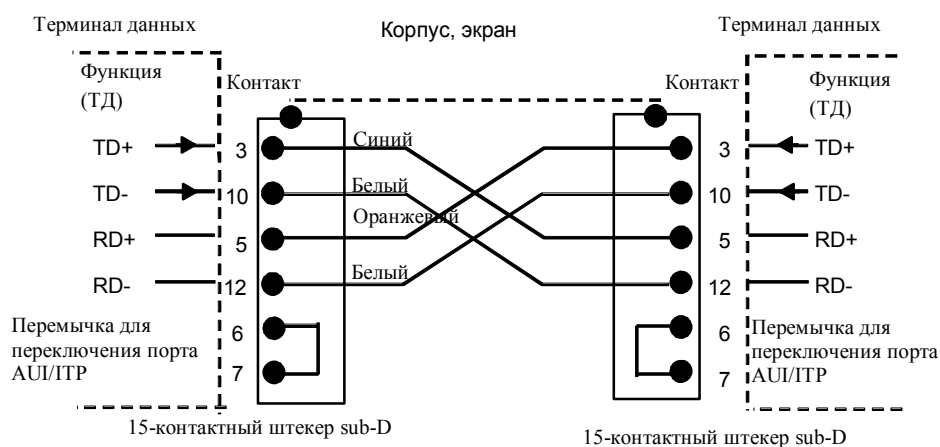
Рисунок 4–6 Разводка контактов стандартной промышленной витой пары
