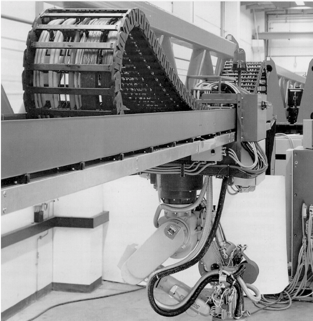
Рисунок 5-4 Пример использования стеклянного волоконно-оптического кабеля для подвижных механизмов в волочащемся шлейфе
