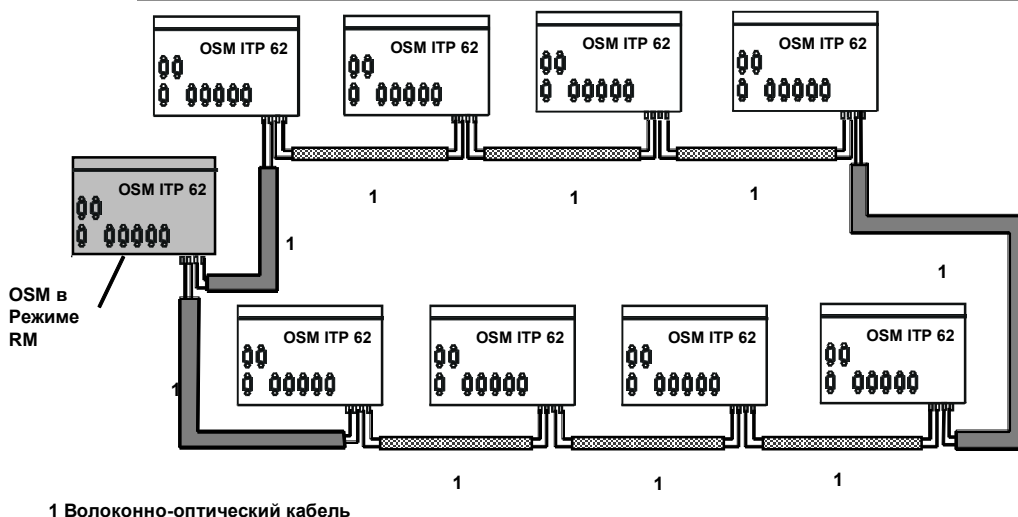
Рисунок 3–11 Резервированное кольцо с использованием модулей OSM
