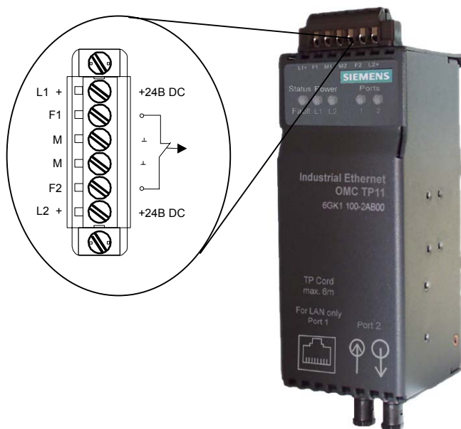
Рисунок 2: Клеммная колодка
