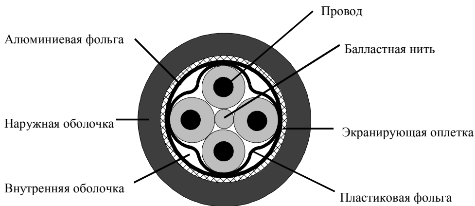
Рисунок 4–3 Вид поперечного сечения витой пары FastConnect (FC)
