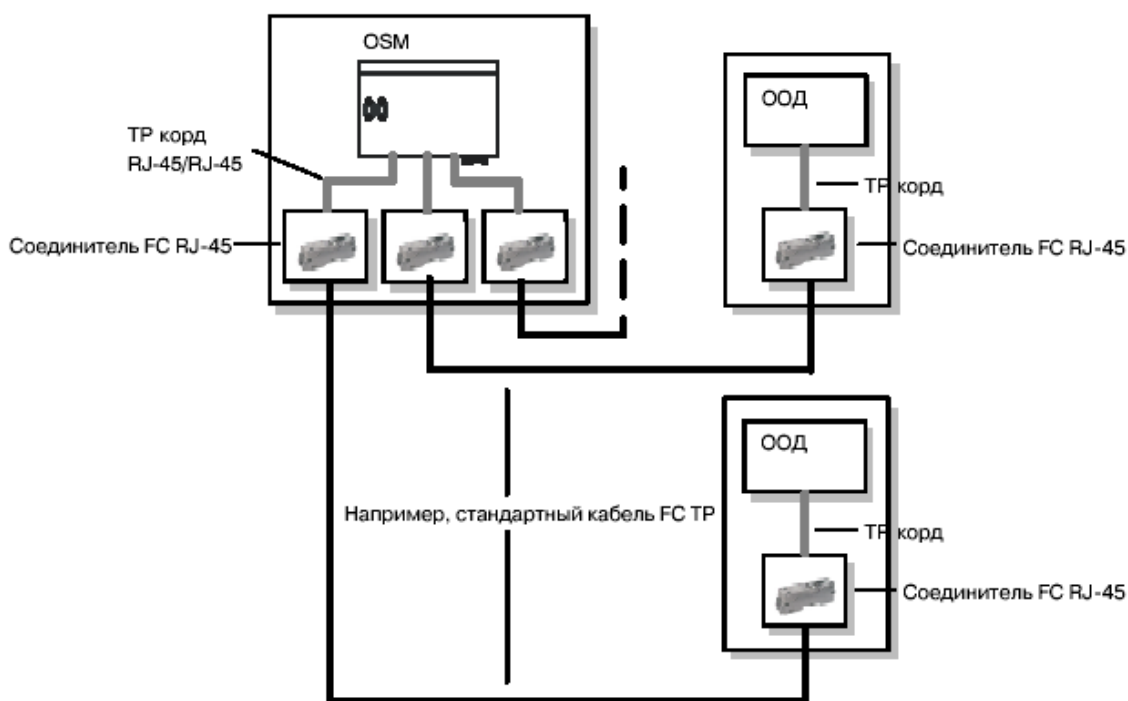
Рисунок 4-21 Конфигурация системы с соединителями FC RJ-45
