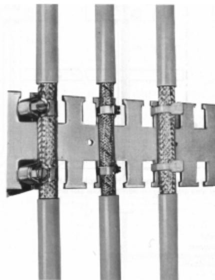
Рисунок 7–3 Обеспечение контакта с экраном по месту ввода в шкаф.
