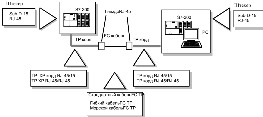
Рисунок 4–12 Кабельная система между двумя терминальными устройствами
