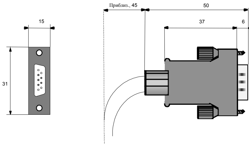
Рисунок 9-12 9-контактный Sub-D штекер для установки пользователем (габариты в мм)
