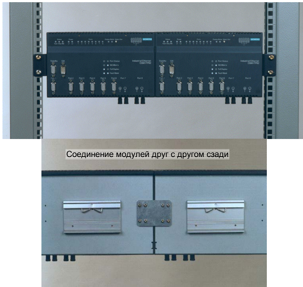
Рисунок 30: Монтаж в 19" шкаф
