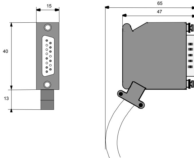
Рисунок 9–14 15-контактный Sub-D штекер для установки пользователем (габариты в мм)
