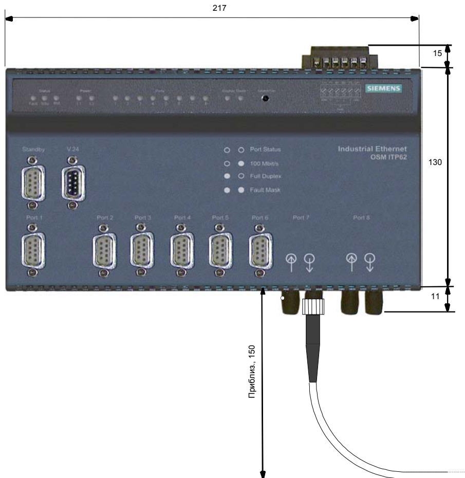
Рисунок 9-2 OSM ITPxx для Industrial Ethernet (габариты в мм)
