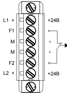
Рисунок 24: Клеммная колодка для цепей питания и сигнального контакта
