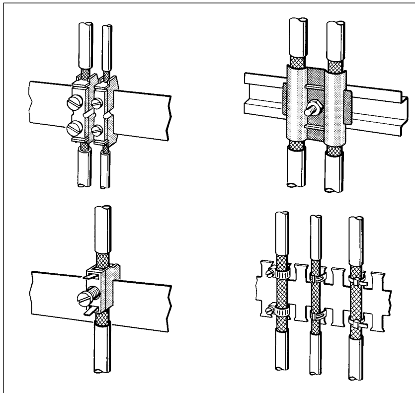
Рисунок 7–2 Крепление экранированных кабелей с помощью кабельных зажимов и стяжек (схематичное представление).
