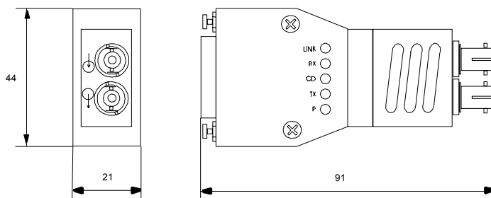
Рисунок 9–10 Оптический трансивер MINI–OTDE (габариты в мм)
