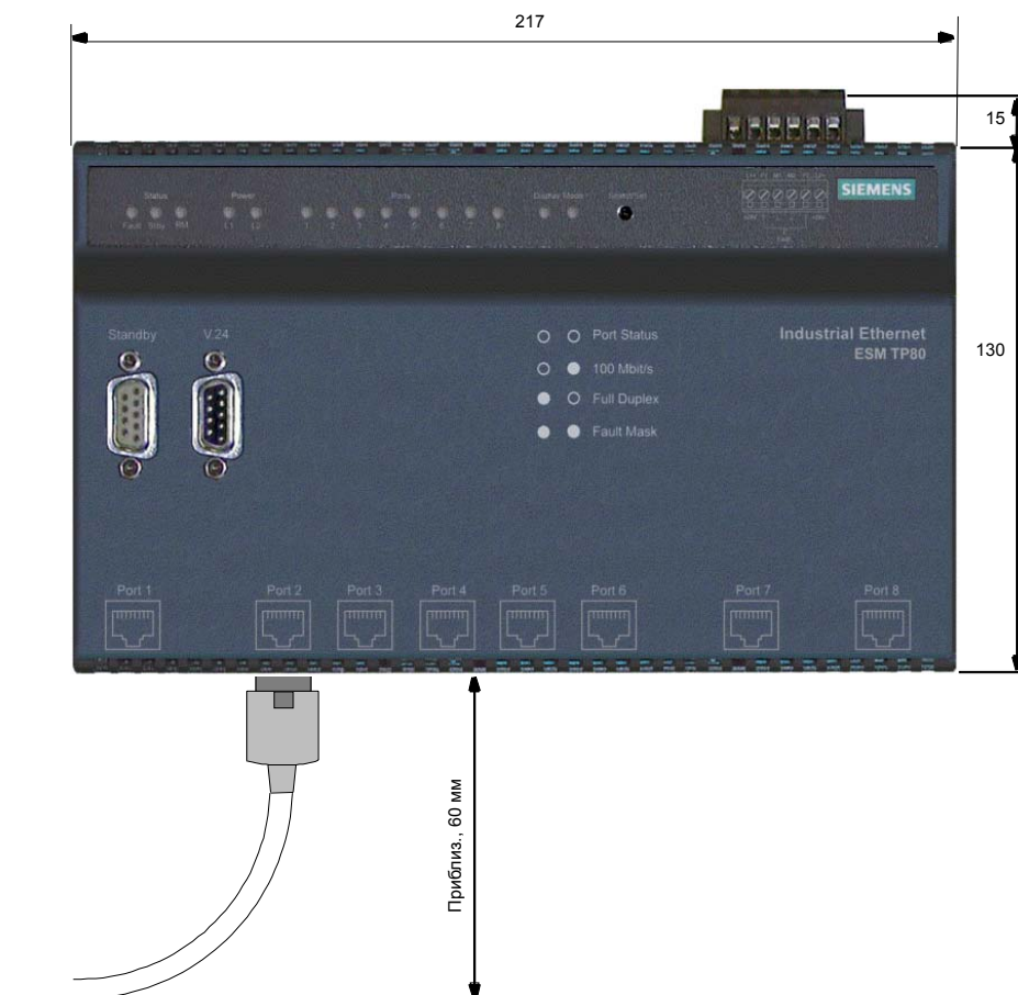
Рисунок 9–6 ESM TP80 для Industrial Ethernet (габариты в мм)
