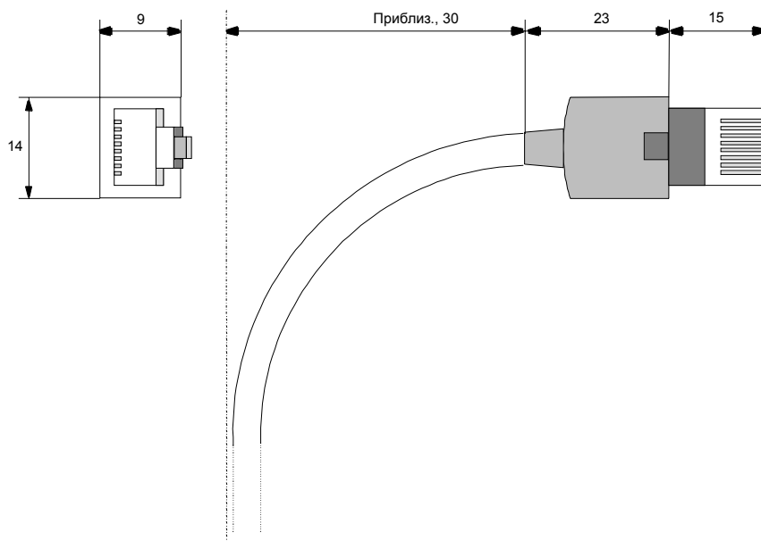
Рисунок 9-16 Штекер RJ-45 (габариты в мм)
