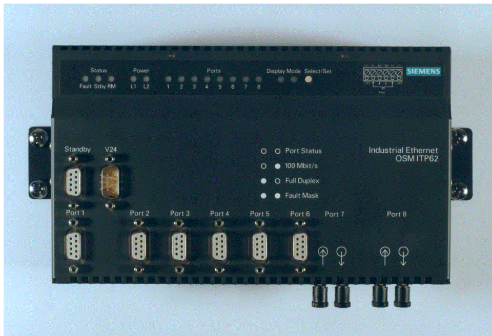
Рисунок 31: Настенный монтаж
