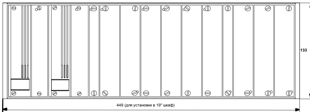
Рисунок 9–8 Активный звездообразный разветвитель ASGE (вид спереди; габариты в мм)
