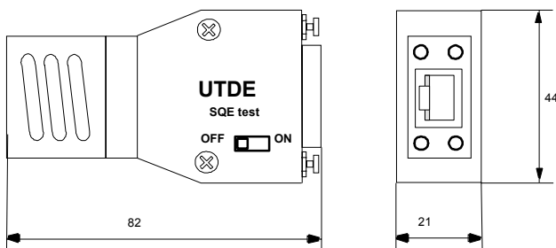
Рисунок 9–11 Электрический трансивер Mini–UTDE RJ–45 (габариты в мм)
