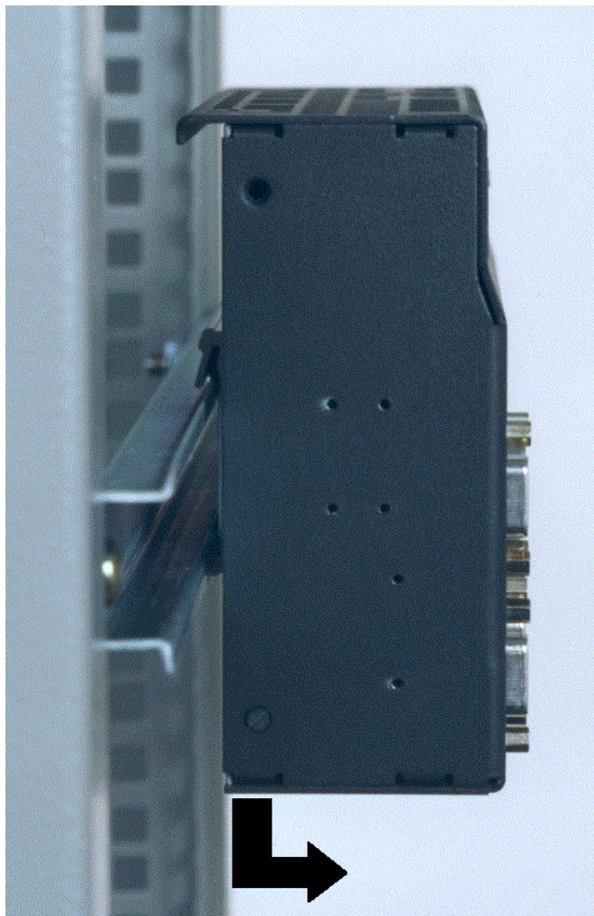
Рисунок 28. Снятие со стандартной рейки
