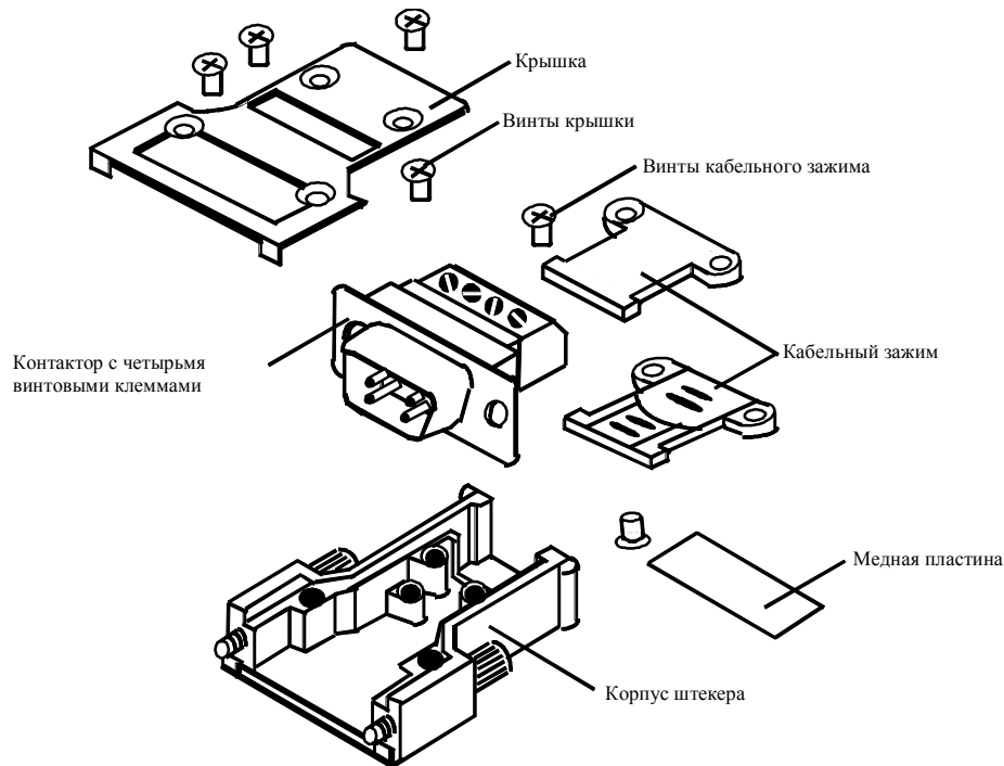
Рисунок 7-7 Sub-D штекер для промышленной витой пары (9-контактный) для монтажа по месту использования
