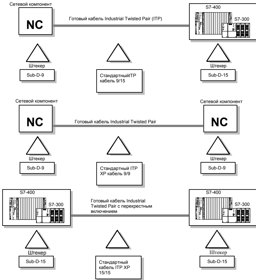
Рисунок 4–5 Использование готовых промышленных витых пар для организации прямых каналов связи между двумя компонентами.
