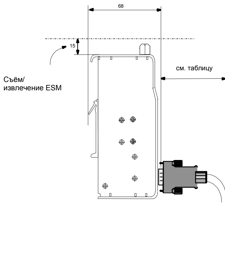
Рисунок 9–7 ESM для Industrial Ethernet (вид сбоку; габариты в мм)
