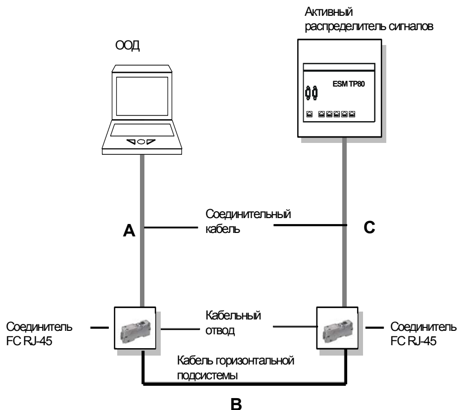
Рисунок 4–1 Конфигурация системы с использованием соединителей FC RJ–45
