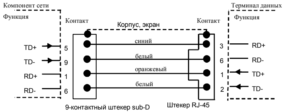
e) Разводка контактов TP корд 9-45/RJ-45
