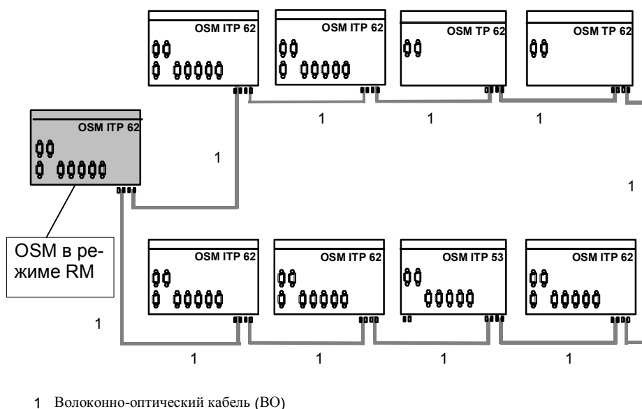
Рисунок 12: Резервированное кольцо с модулями OSM
