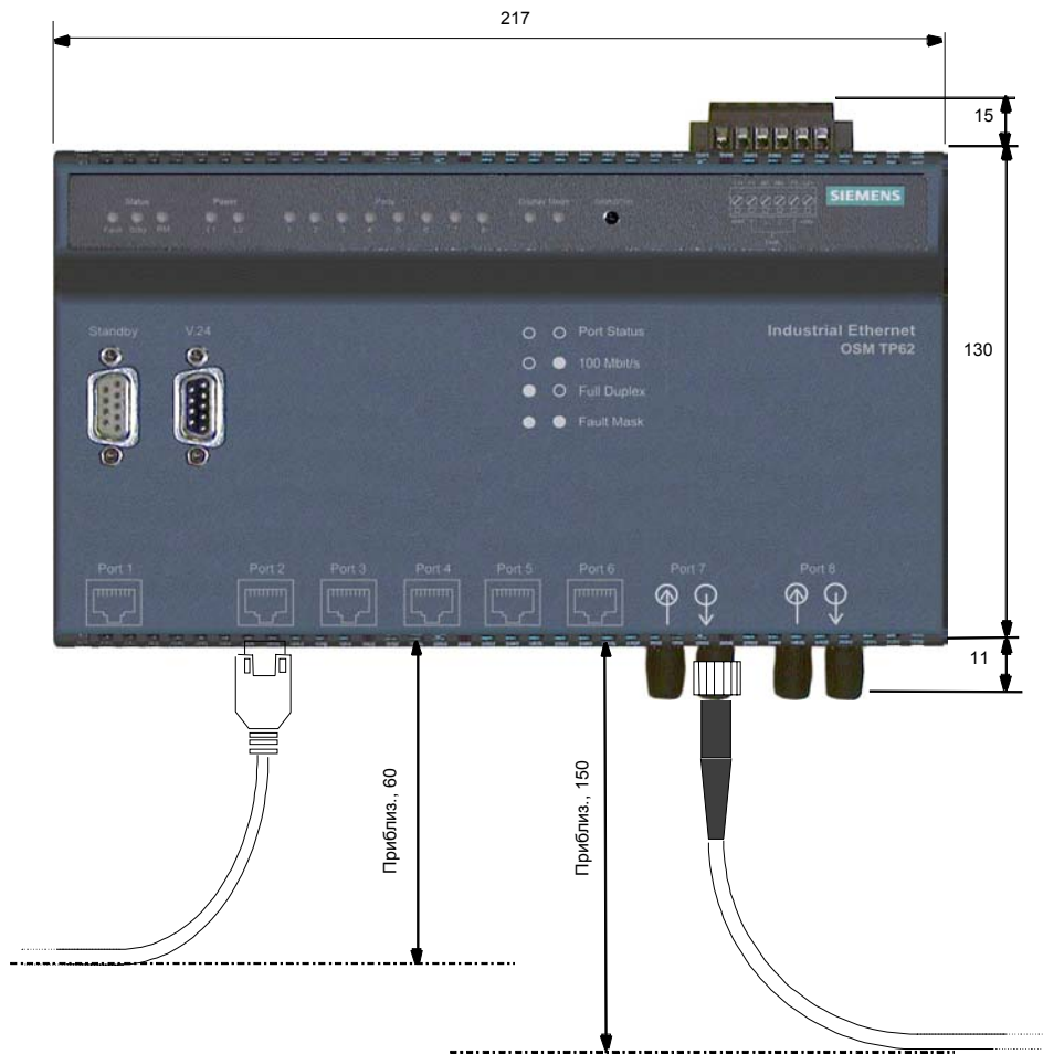
Рисунок 9-3 OSM TPxx для Industrial Ethernet (габариты в мм)
