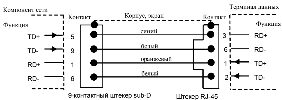
c) Разводка контактов TP корд 9/RJ-45
