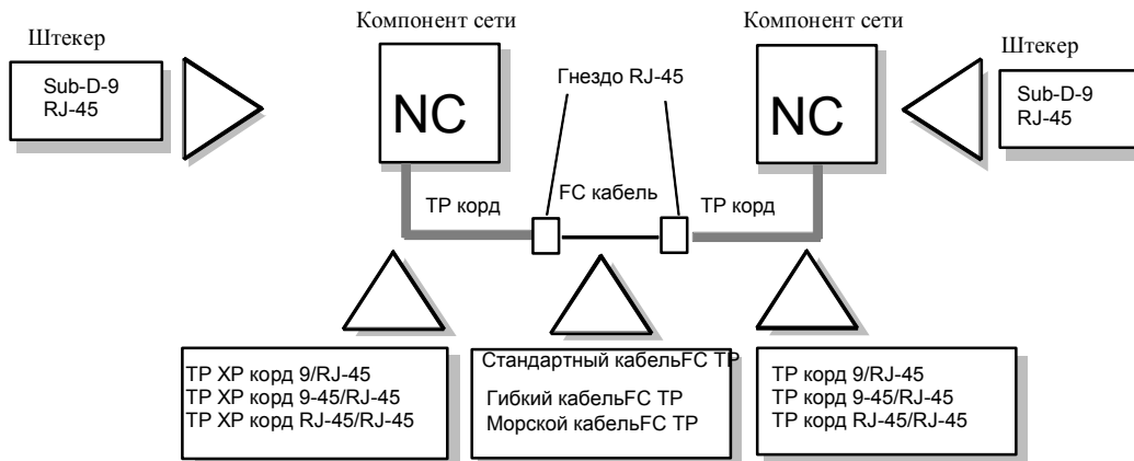
Рисунок 4–11 Структурированная кабельная система между двумя компонентами сети
