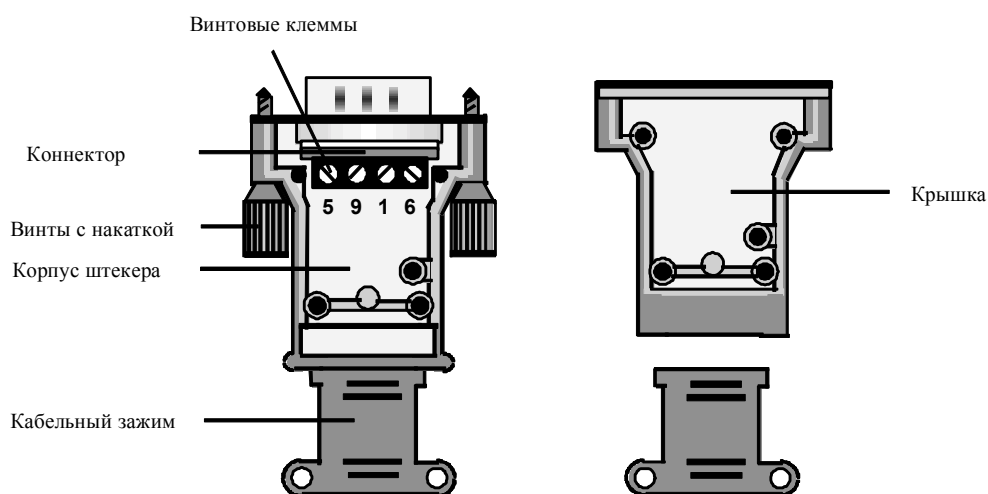
Рисунок 4–17 Штекер sub-D для промышленной витой пары (9-контактный) для монтажа по месту использования
