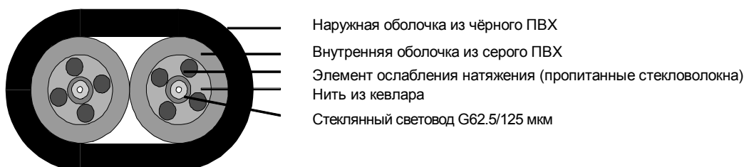
Рисунок 5-1 Структура стандартного волоконно-оптического кабеля
