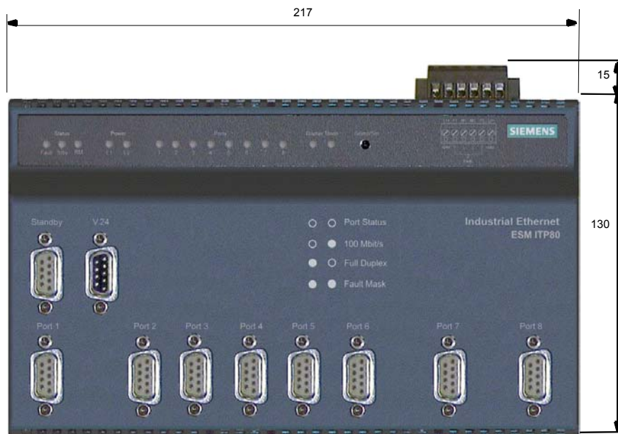
Рисунок 9–5 ESM ITP80 для Industrial Ethernet (габариты в мм)
