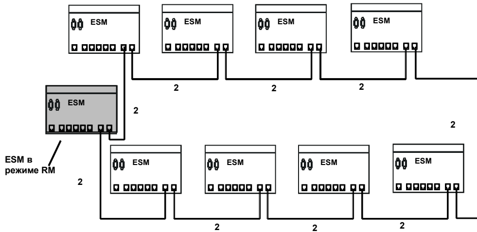
2 Структура кабельных соединений с использованием витой пары SIMATIC NET
