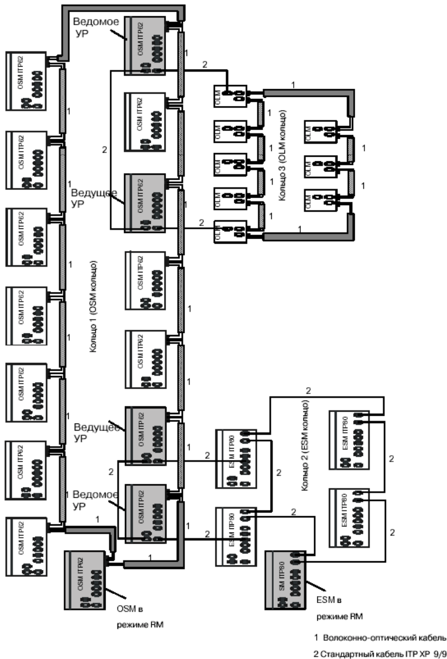
Рисунок 3–12 Объединение сегментов сети с целью резервирования
