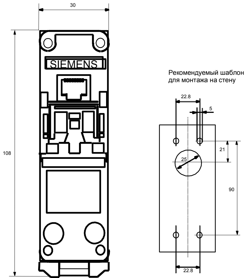
Рисунок 9-17 Соединитель RJ-45 IE FC (габариты в мм)
