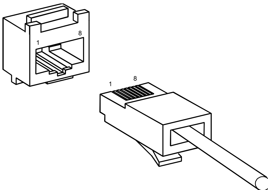
Рисунок 4-19 Гнездо и вилка RJ-45
