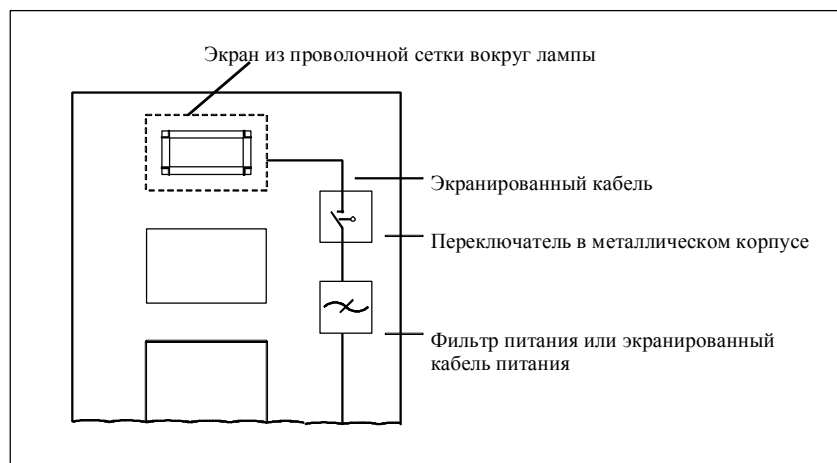
Рисунок 7-4 Меры по подавлению помех от ламп дневного света в шкафу.
