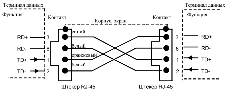
b) Разводка контактов TP XP корда RJ-45/RJ-45
