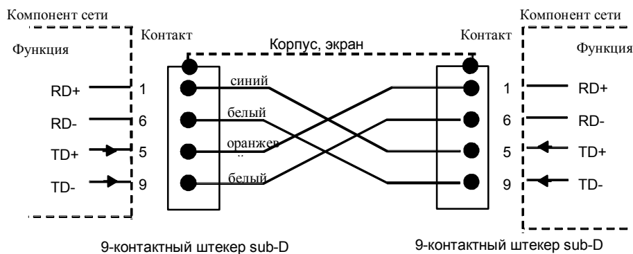
г) Разводка контактов ТР ХР кабеля 9/9
