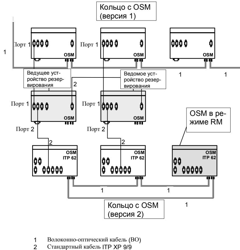
Рисунок 18: Резервное объединение колец с модулем OSM V1 в качестве ведущего/ведомого устройства резервирования
