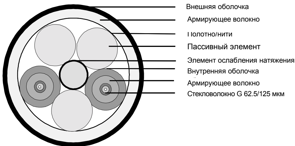
Рисунок 5-3 Структура гибкого волоконно-оптического кабеля для подвижных механизмов
