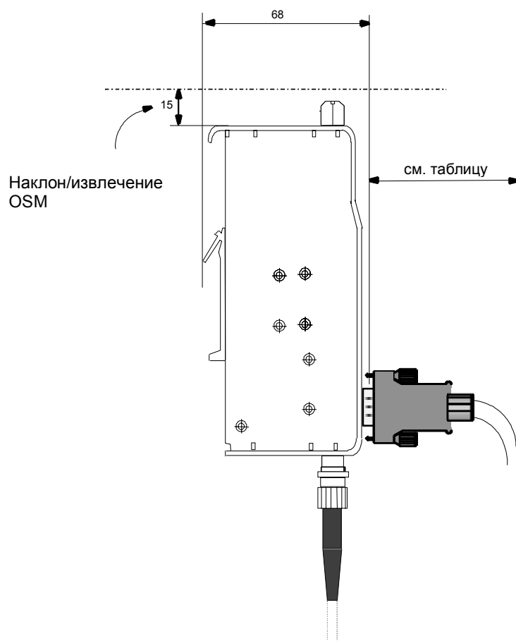
Рисунок 9-4 OSM для Industrial Ethernet (вид сбоку; габариты в мм)
