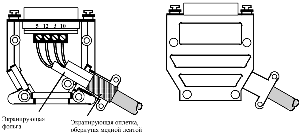
Рисунок 7–10 15-контактный sub-D штекер, смонтированный на стандартный кабель
