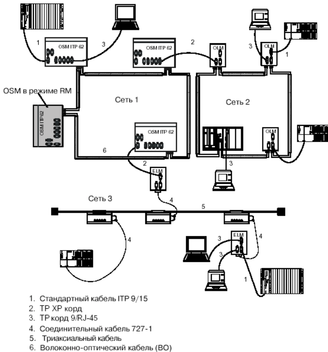
Рисунок 2–2 Структура сети с использованием сетевых компонентов Industrial Ethernet
