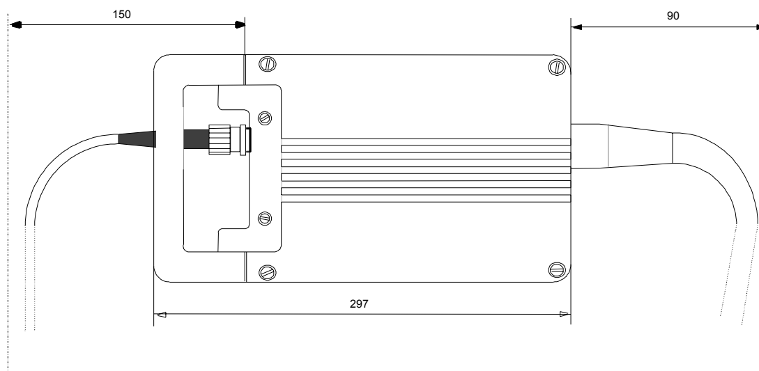
Рисунок 9–9 Активный звездообразный разветвитель ASGE (вид сбоку; габариты в мм)
