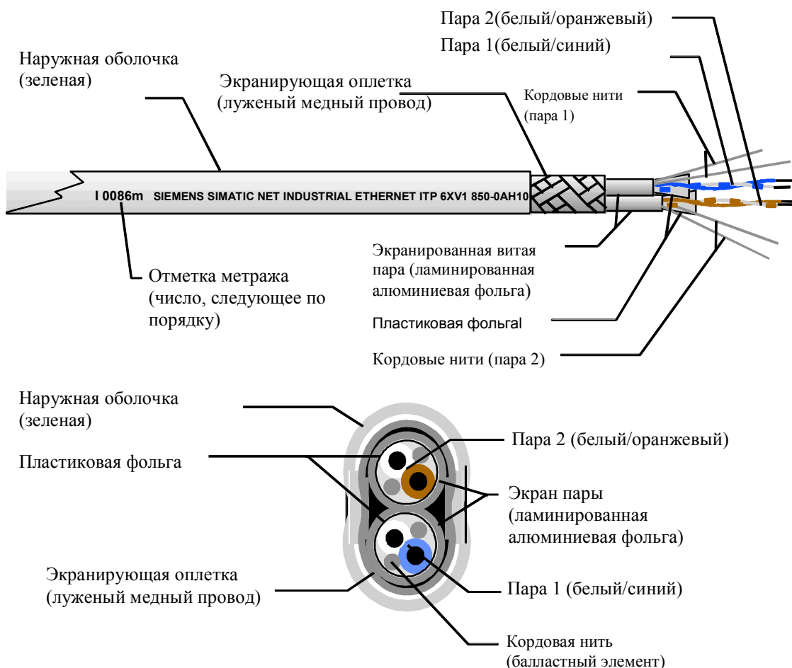
Рисунок 4–2 Структура стандартной промышленной витой пары
