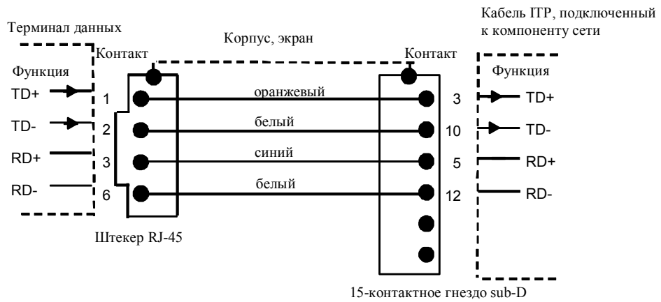
Рисунок 4–16 Разводка контактов кабеля/переходника TP 15/RJ–45
