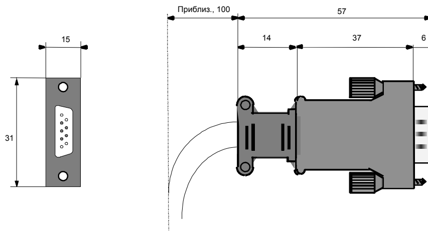
Рисунок 9-12 9-контактный Sub-D штекер для установки пользователем (габариты в мм)
