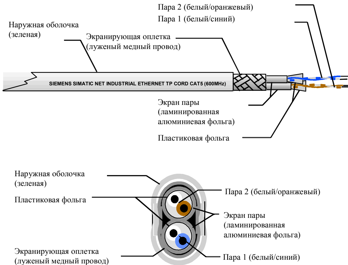
Рисунок 4–4 Структура TP корда (PIMF)
