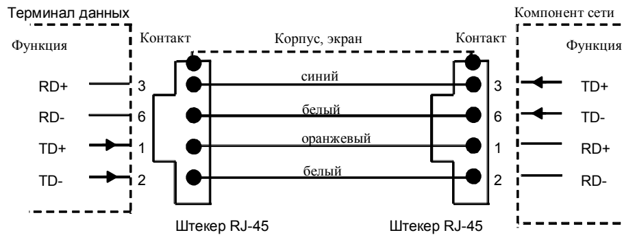
a) Разводка контактов TP корда RJ-45/RJ-45
