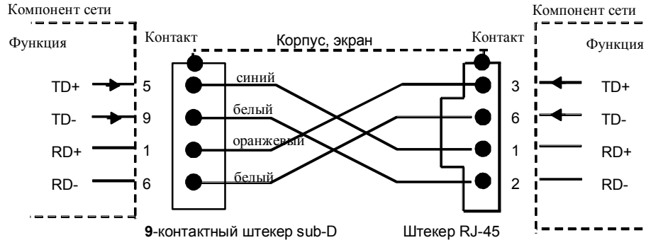
d) Разводка контактов TP XP корда 9/RJ-45
