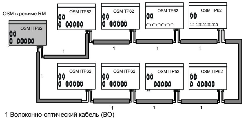
Рисунок 6–9 Резервированное кольцо с использованием OSM
