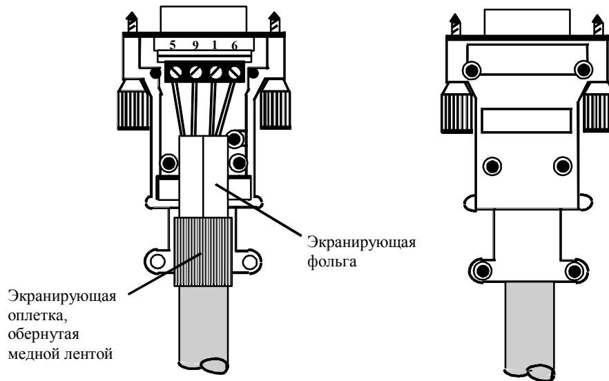
Рисунок 7–8 9-контактный sub-D штекер (вилка), смонтированный на стандартный кабель
