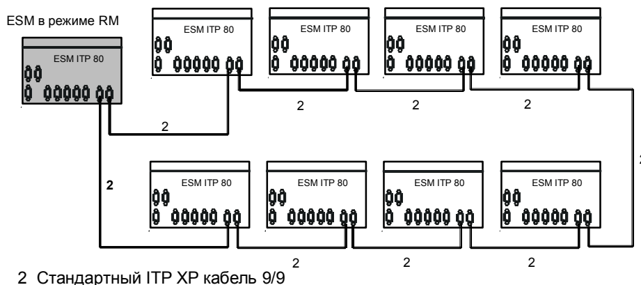
Рисунок 6–10 Резервированное кольцо с использованием ESM
