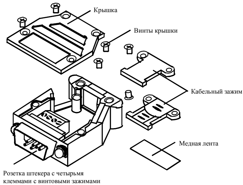
Рисунок 7–9 15-контактный sub-D штекер для монтажа по месту использования
