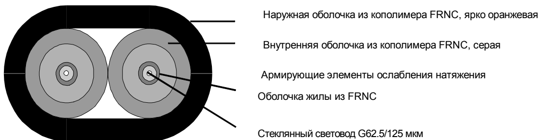
Рисунок 5-2 Структура волоконно-оптического кабеля INDOOR
