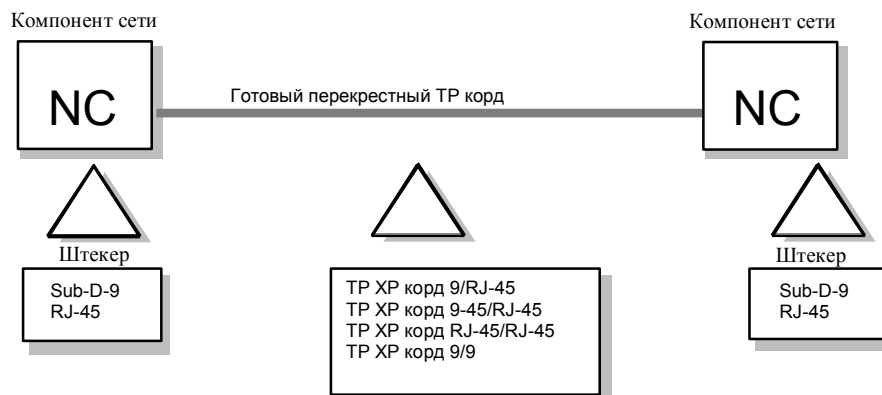
Рисунок 4–8 Прямая связь двух компонентов сети
