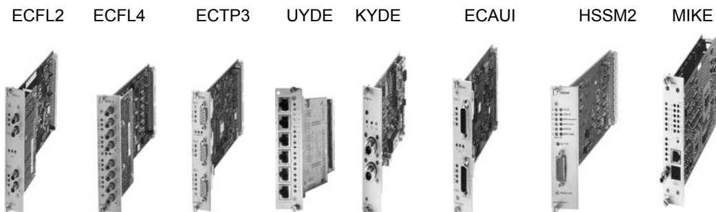
Рисунок 6–15 Интерфейсные карты для звездообразного разветвителя ASGE
