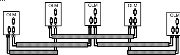
Рисунок 3–6 Вариант кабельных соединений для сетевой структуры с топологией оптического резервированного кольца
