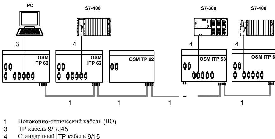
Рисунок 10: Шина с применением OSM
