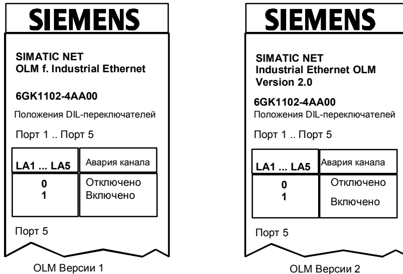
Рисунок 6–3 Таблички с указанием версий для OLM Версии 1 и Версии 2.0
