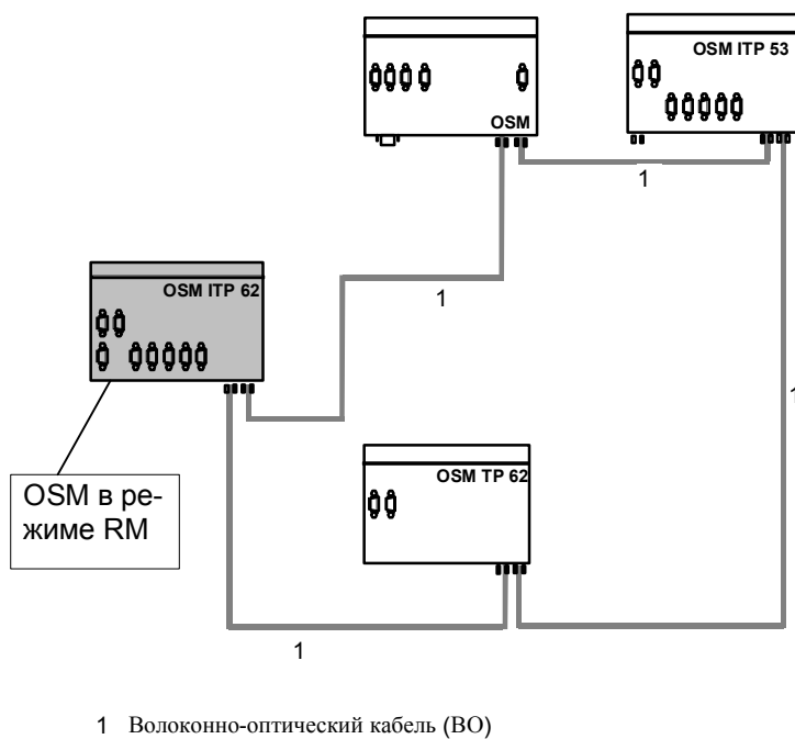
Рисунок 17: Кольцо с модулем OSM (версия 2) в качестве устройства управления резервированием
