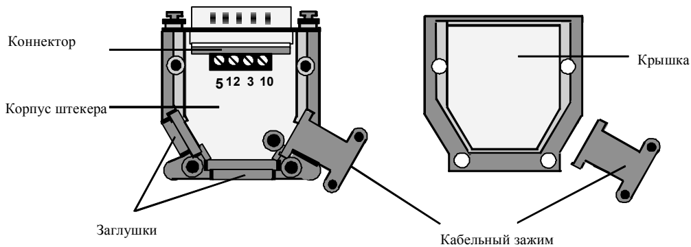
Рисунок 4–18 Штекер sub-D для промышленной витой пары (15-контактный) для монтажа по месту использования
