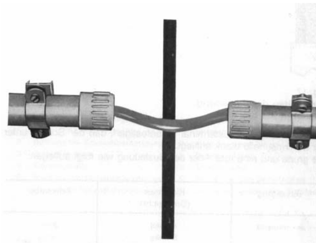
Рисунок 7–6 Прерывание кабелепровода на стыке
