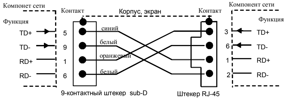
f) Разводка контактов TP XP корд 9-45/RJ-45
