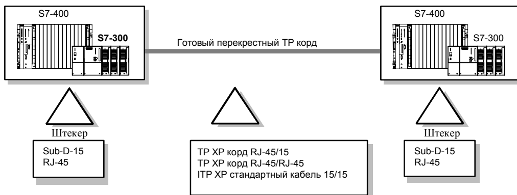
Рисунок 4–9 Прямая связь между двумя терминальными устройствами
