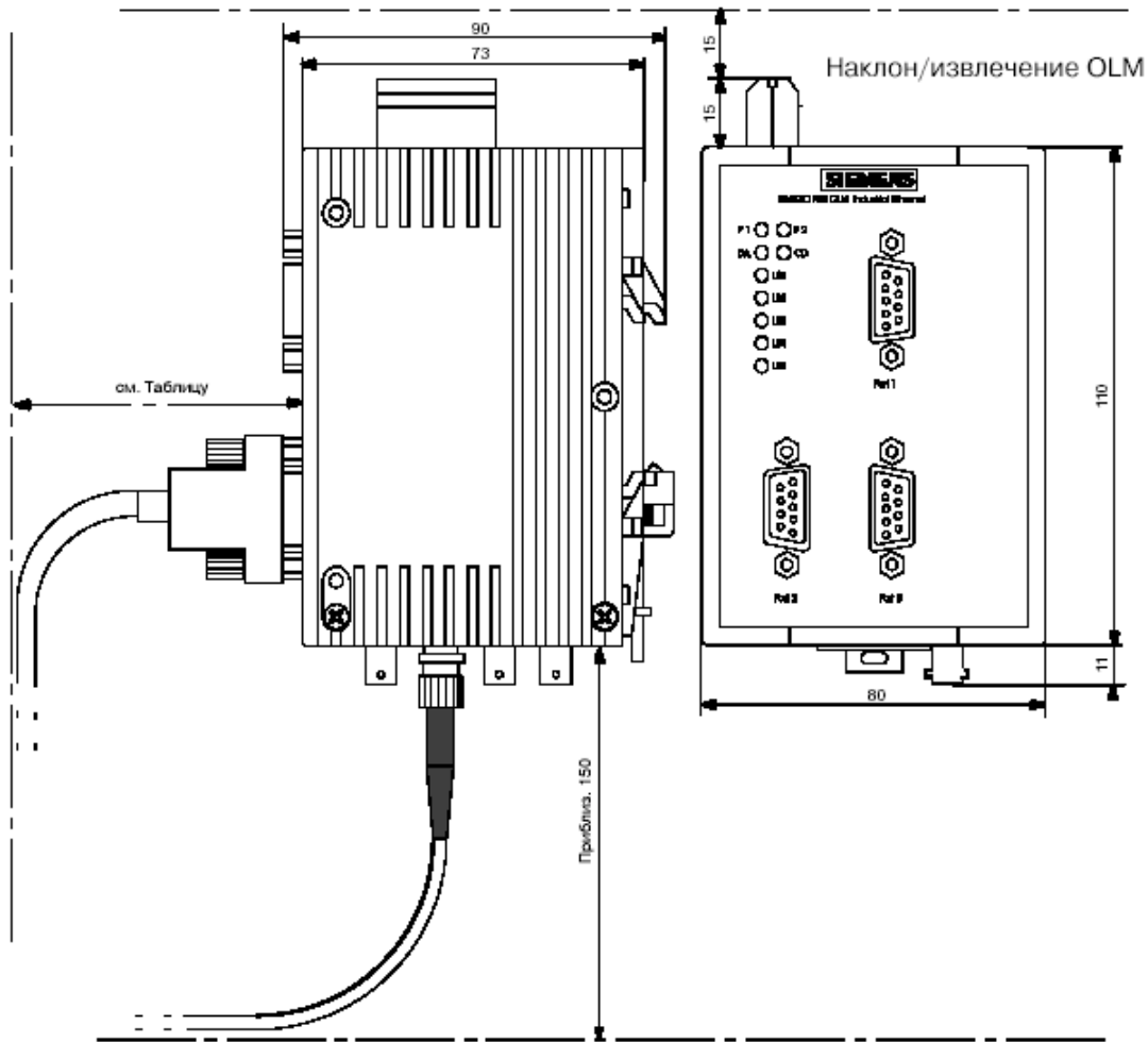
Рисунок 9–1 OLM/ELM для Industrial Ethernet (габариты в мм)
