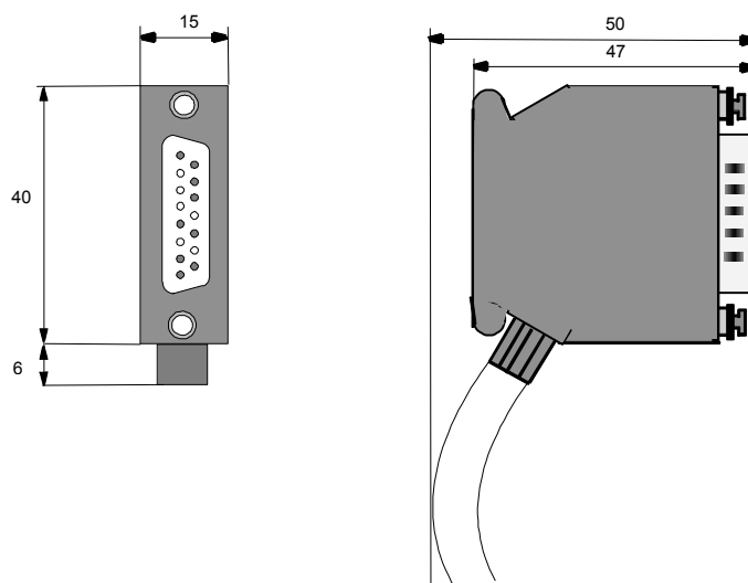
Рисунок 9–14 15-контактный Sub-D штекер для установки пользователем (габариты в мм)
