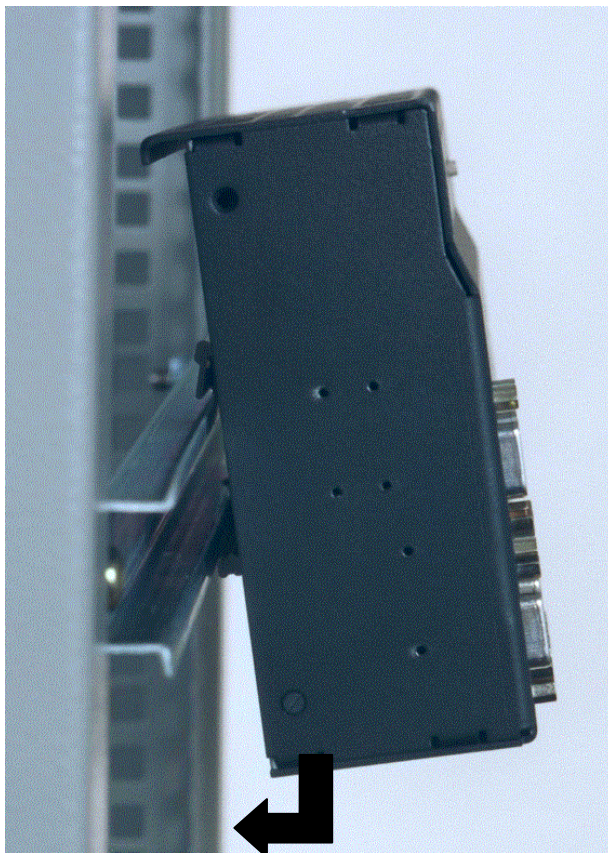
Рисунок 27: Монтаж OSM на стандартную DIN-рейку
