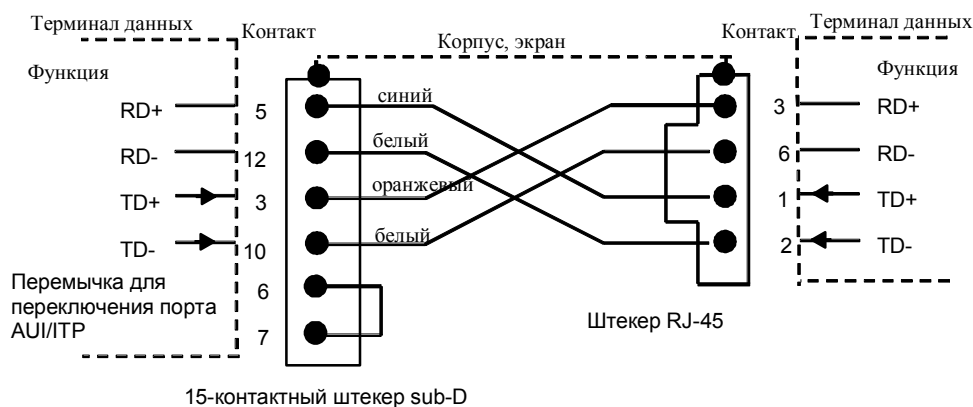
и) Разводка контактов ТР ХР кабеля 15/RJ-45
