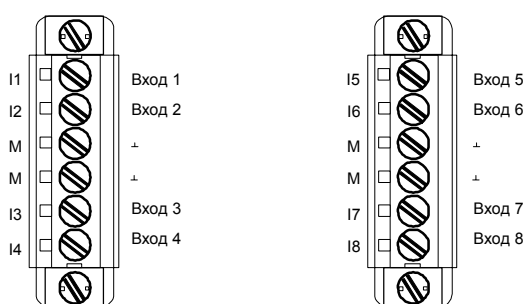
Рисунок 25: Клеммные колодки для подключения дискретных входных сигналов
