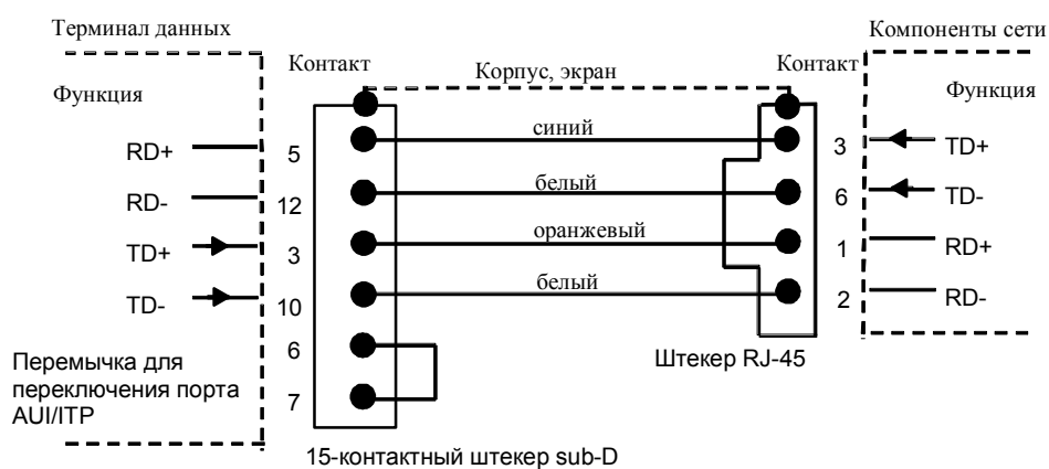
h) Разводка контактов ТР кабеля 15/RJ-45
