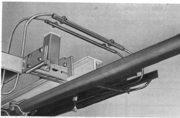
Рисунок 7–5 Механическая защита кабеля ЛС
