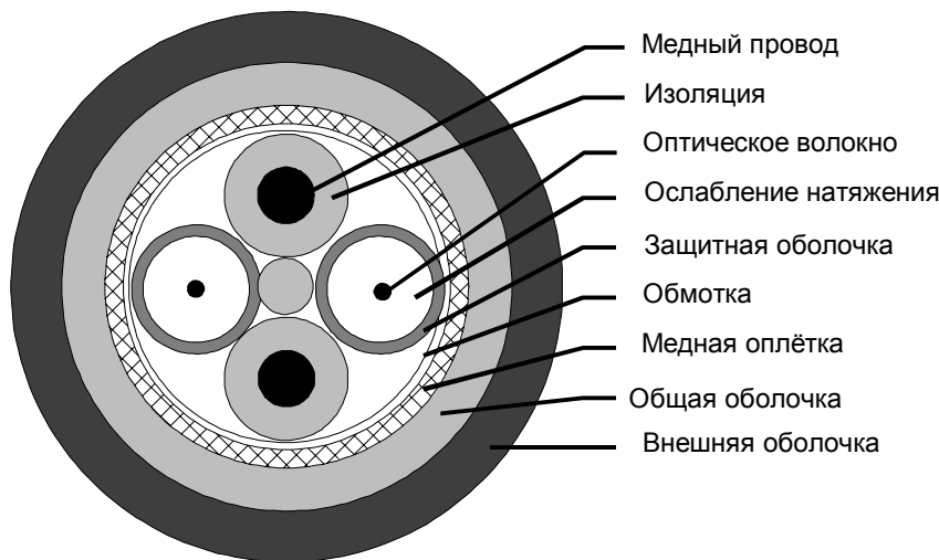
Рисунок 5-5 Структура дуплексного волоконно-оптического судового кабеля SIENOPYR
