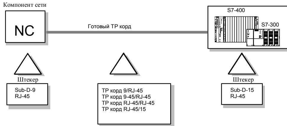
Рисунок 4–7 Прямая связь ООД с компонентом сети
