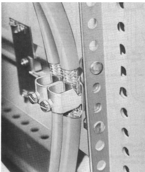
Рисунок 7–3 Обеспечение контакта с экраном по месту ввода в шкаф.
