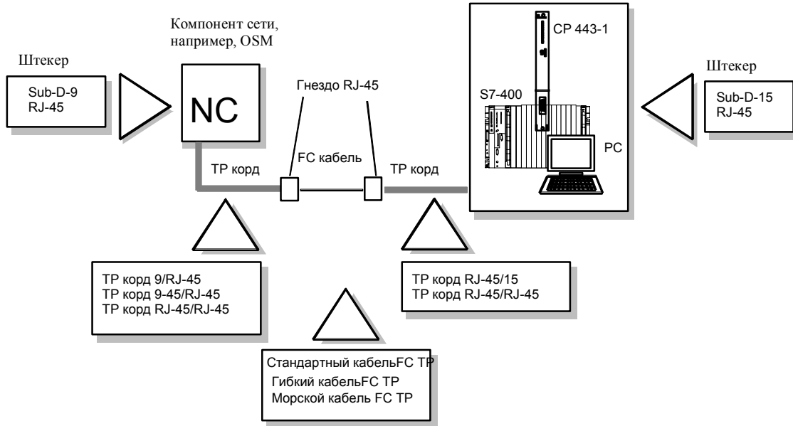
Рисунок 4–10 Структурированная кабельная система между ООД и компонентом сети
